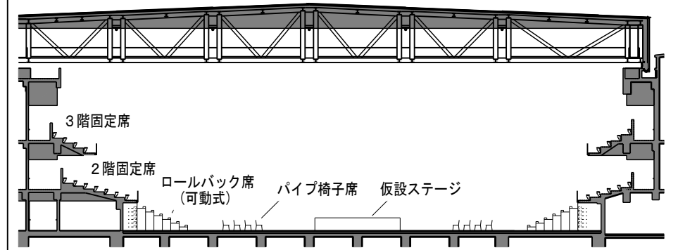
断面図(センターステージ形式)
